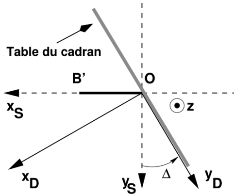
Figure 3 : Cadran vertical déclinant.
