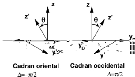
Figure 5 : Disposition des repères pour le cadran occidental et oriental.
