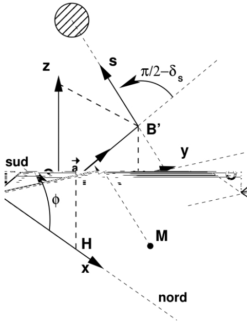
Figure 1 : Schéma du cadran solaire horizontal.
