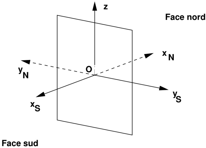
Figure 2 : Cadran verticaux et systèmes de coordonnées associés.
