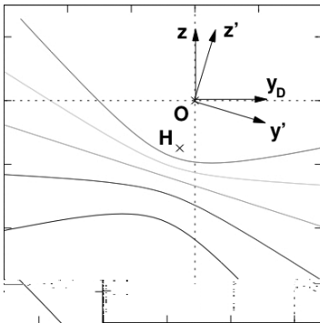
Figure 4a : Cadran vertical de déclinaison - 30° Est pour la latitude \phi = 48^\circ Nord.
