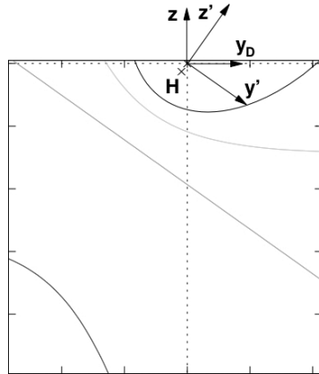
Figure 4b : Cadran vertical de déclinaison - 11° Est pour la latitude \phi = 15^\circ Nord.
